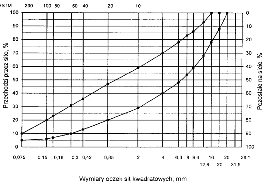
Rys. 1. Krzywe graniczne uziarnienia mieszanki mineralnej BA od 0 do 20 mm do warstwy ścieralnej nawierzchni drogi o obciążeniu ruchem dla KR2
